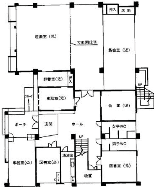
1階平面図
